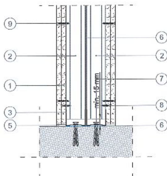
Rys. 9 - przekrój pionowy, połączenie dolne
