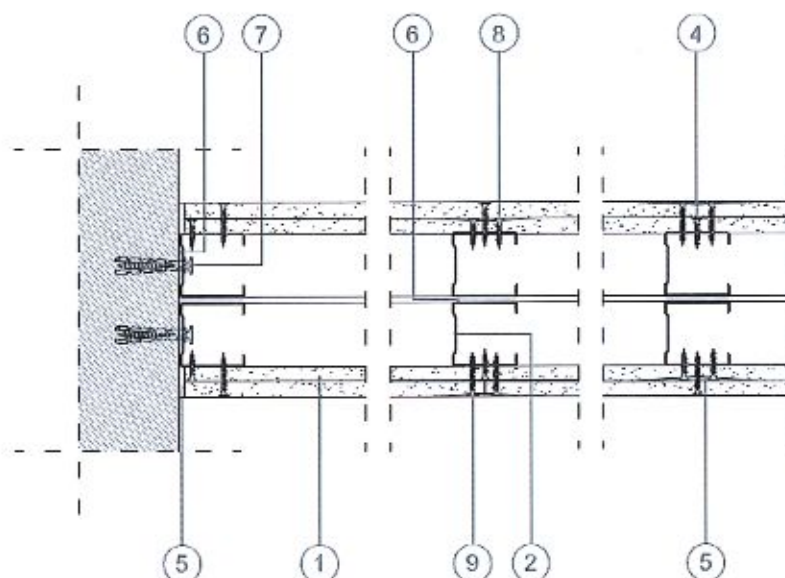
Rys. 10 - przekrój poziomy
