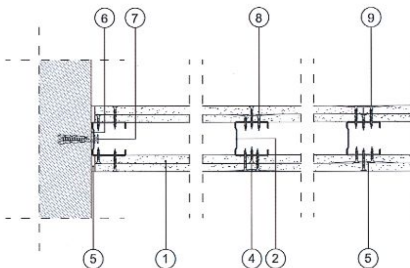
Rys. 4 - przekrój poziomy
