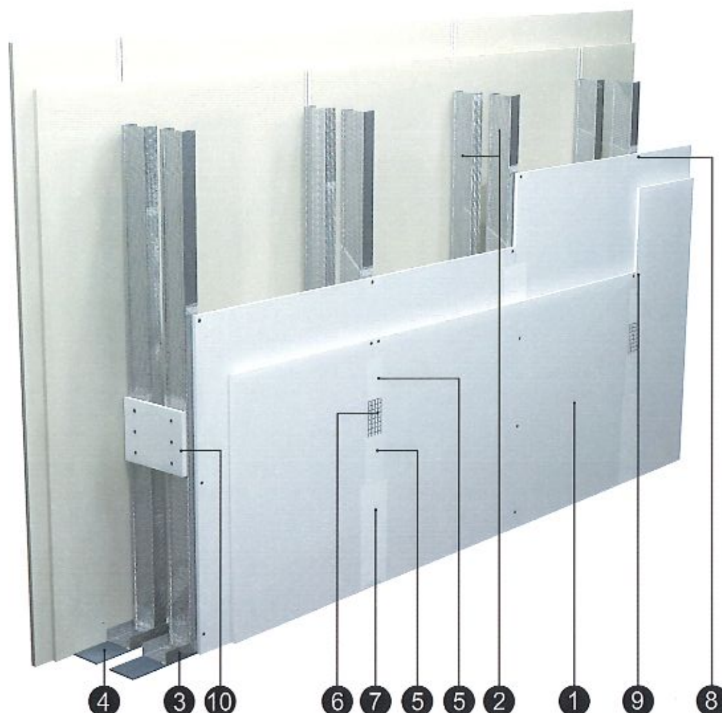
Rys. 13 – widok ściany
