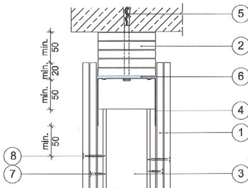
Rys. 18 – przekrój pionowy Połączenie teleskopowe ściany dla ugięcia stropu do 50 mm ze stropem nierozprzestrzeniającym ognia
