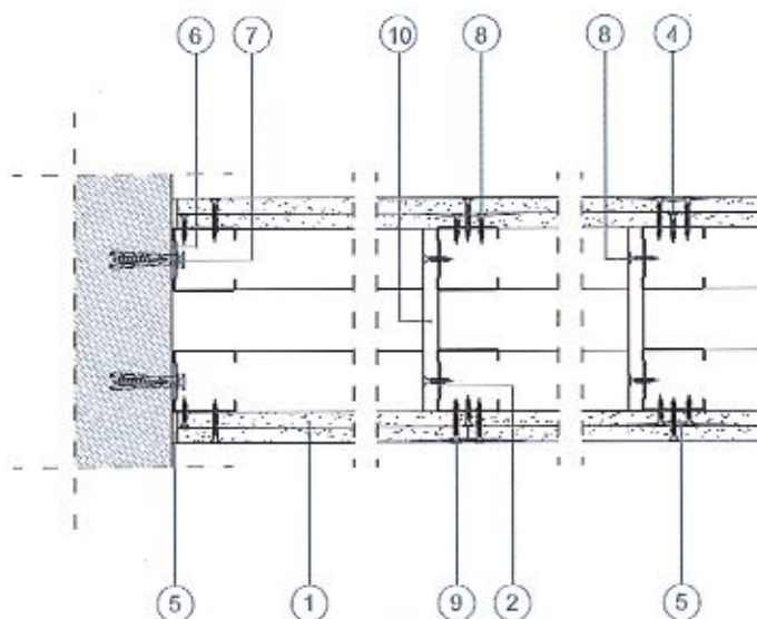
Rys. 16 - przekrój poziomy
