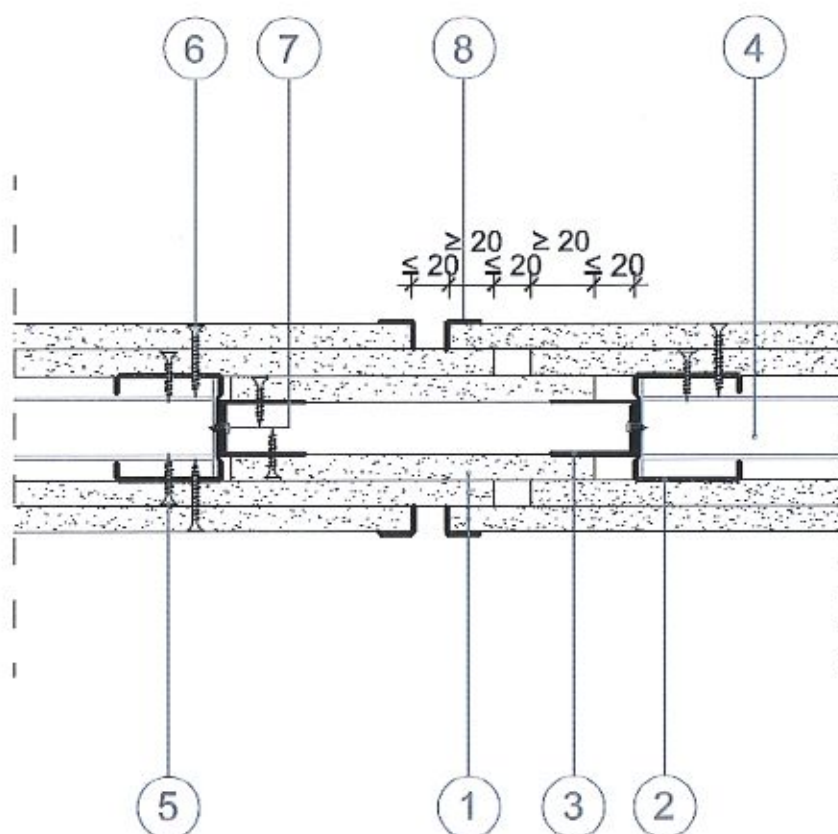
Rys. 5 – połączenie dylatacyjne
