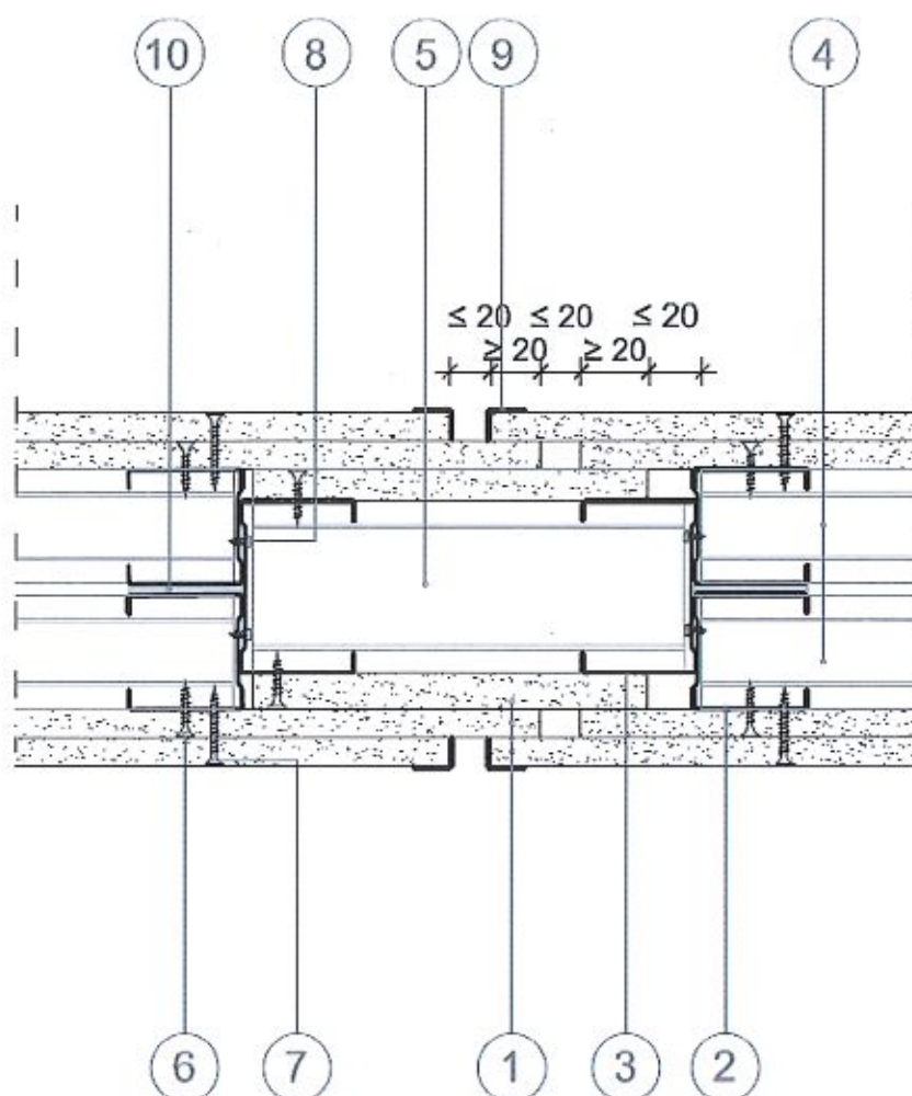
Rys. 11 – połączenie dylatacyjne
